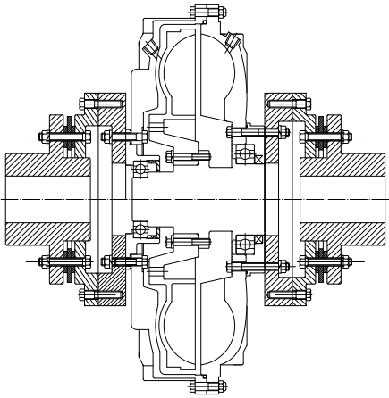
配膜片联轴器型
