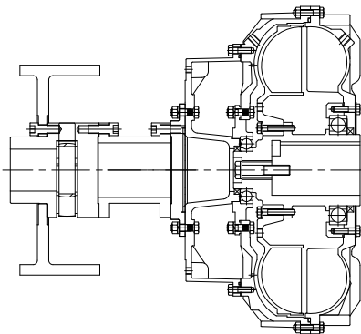
带制动轮可更换弹性体型
