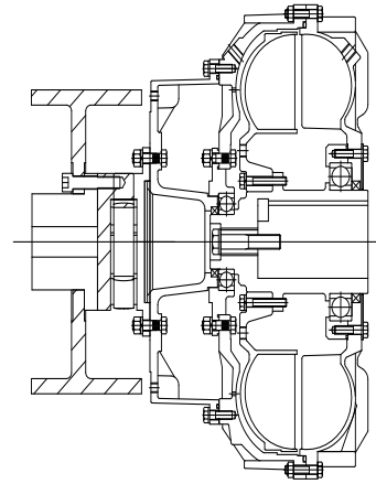
CHCJ-BW带制动轮型
