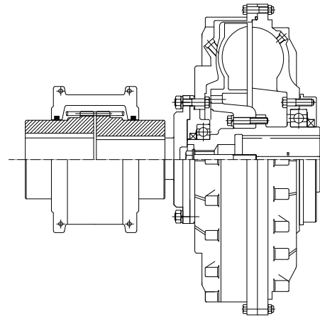
配蛇簧联轴器型
