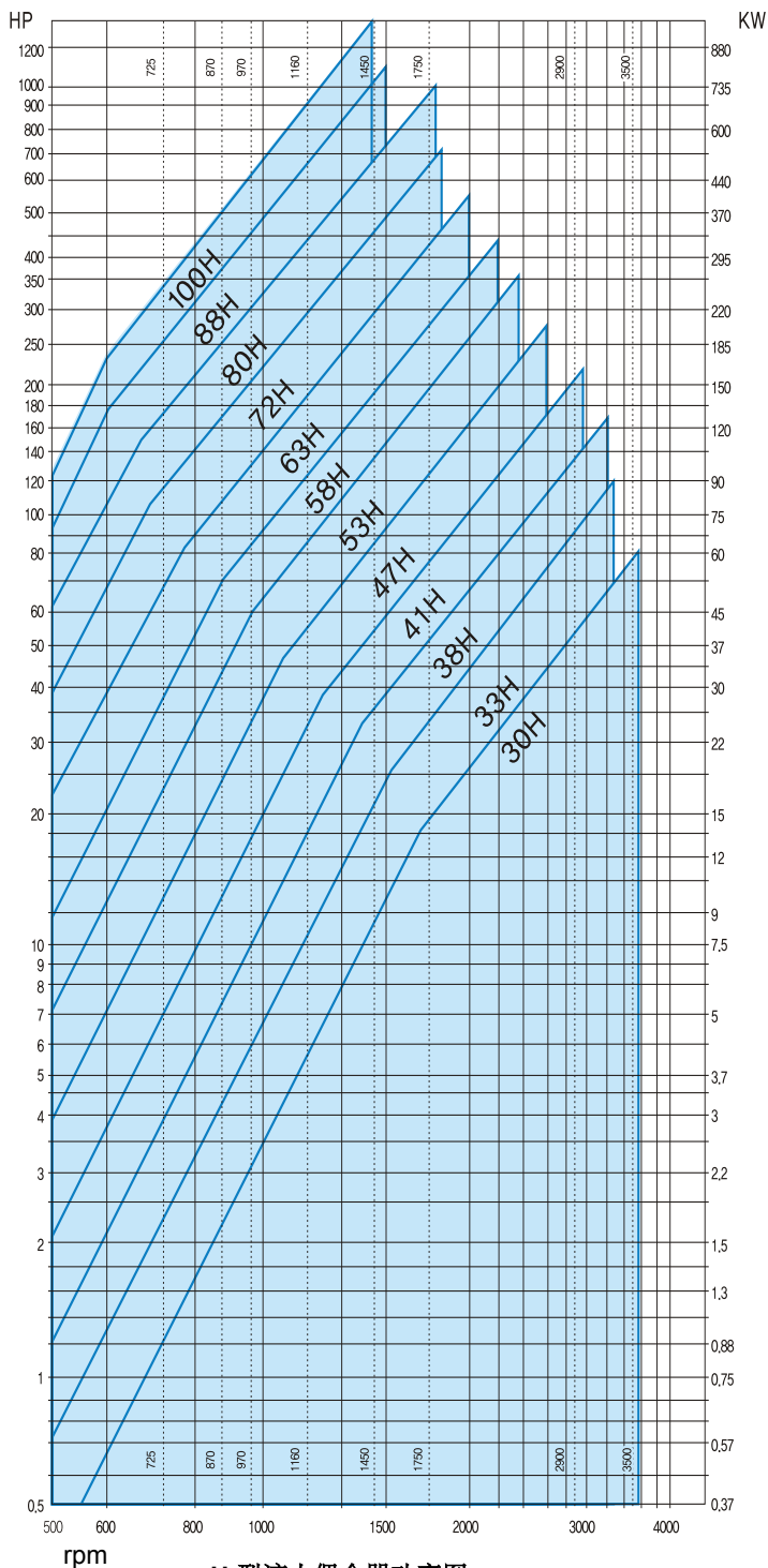
H 型液力偶合器功率图
